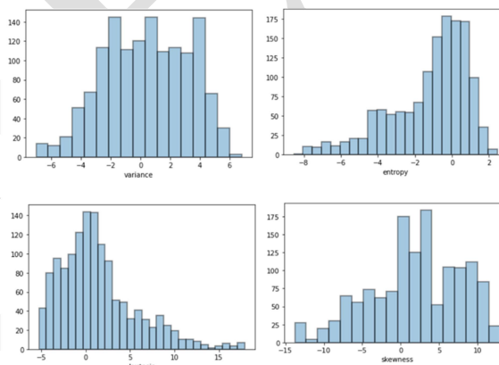
Fig.4 scaling dataset
