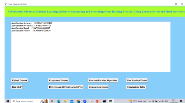
Fig.7.4 Auto Encoder
